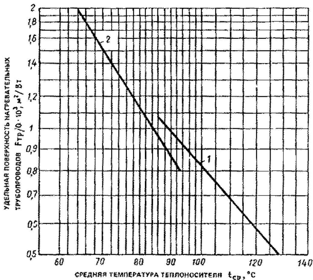
Рис. 13. График для определения требуемой поверхности нагревательных трубопроводов
