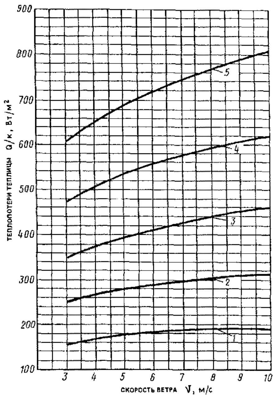
Рис. 12. График для определения теплотерь теплицы
