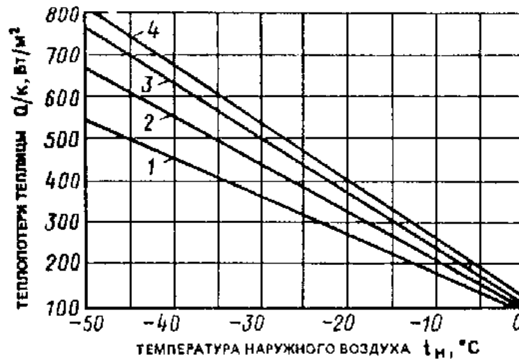
Рис. 14. График для определения теплопотерь теплицы с оребренными трубами системы обогрева
