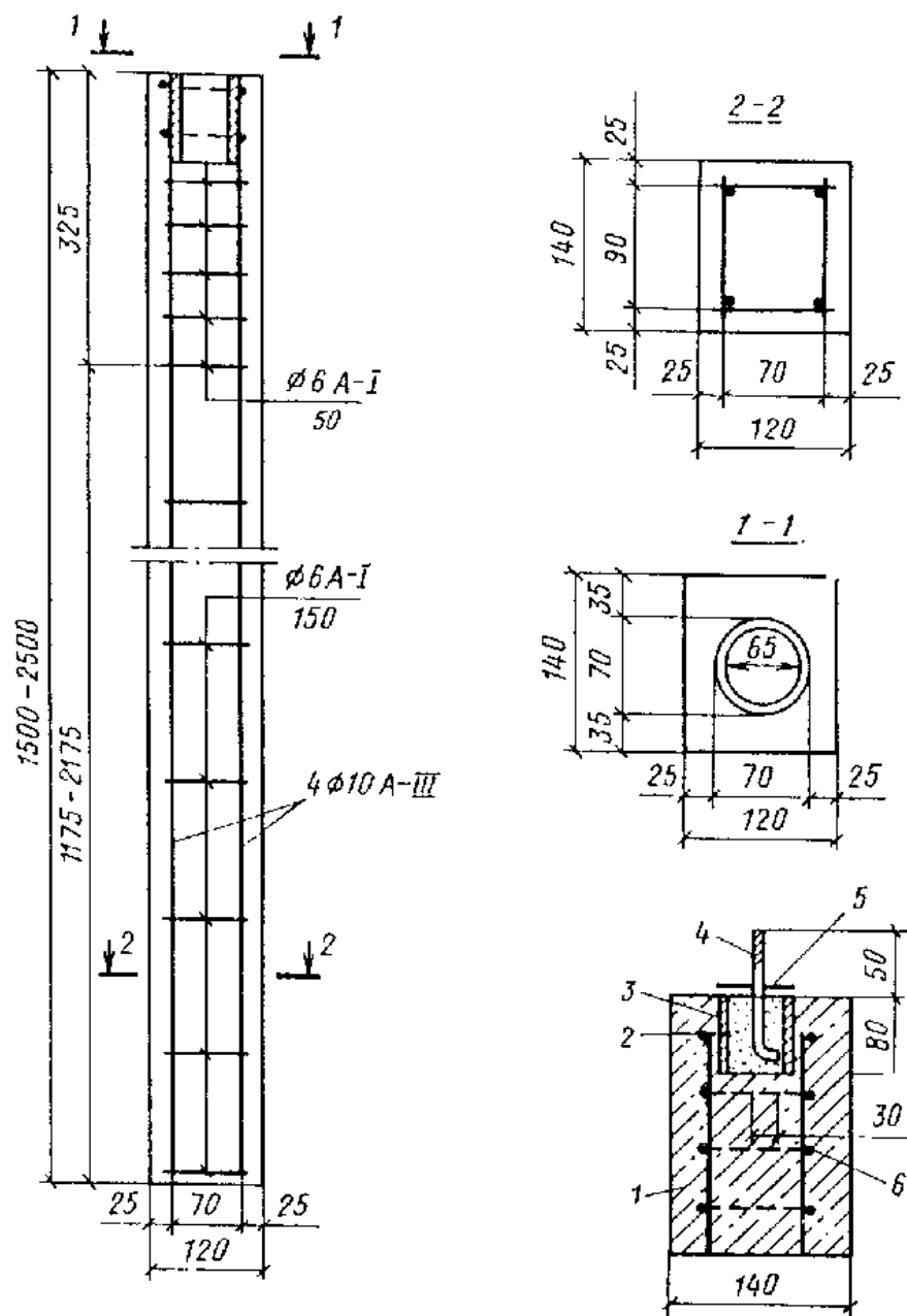
Рис. 1. Пример конструктивного решения свайного фундамента
