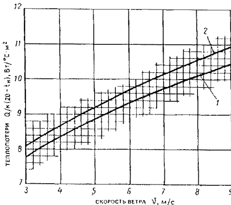
Рис. 21. График для определения теплотерь теплицы с комбинированной системой обогрева при максимальной мощности калориферного обогрева
