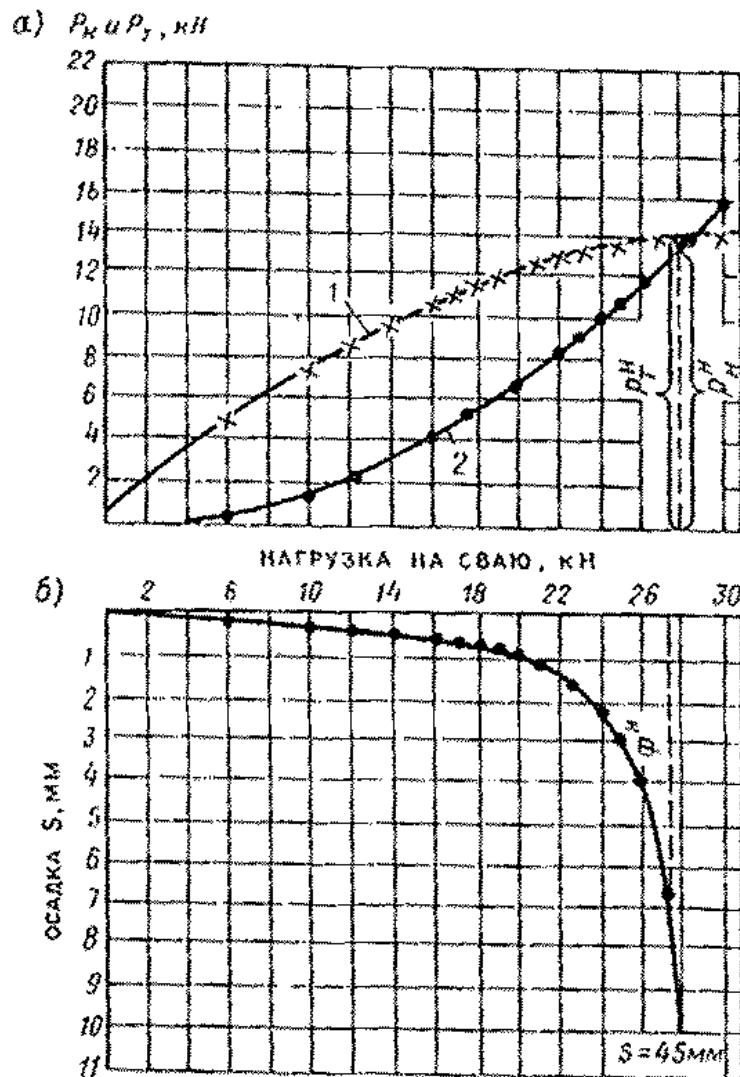
Рис. 5. Графики по результатам испытания сваи - штампа на вертикальную нагрузку
