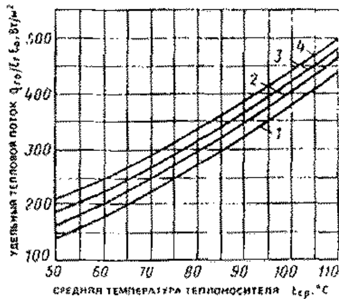
Рис. 17. График для определения удельного теплового потока излучением от гладкой трубы на ограждения
