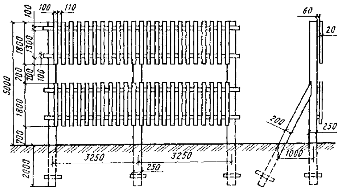
Рис. 29. Деревянный забор с разреженной обрешеткой
