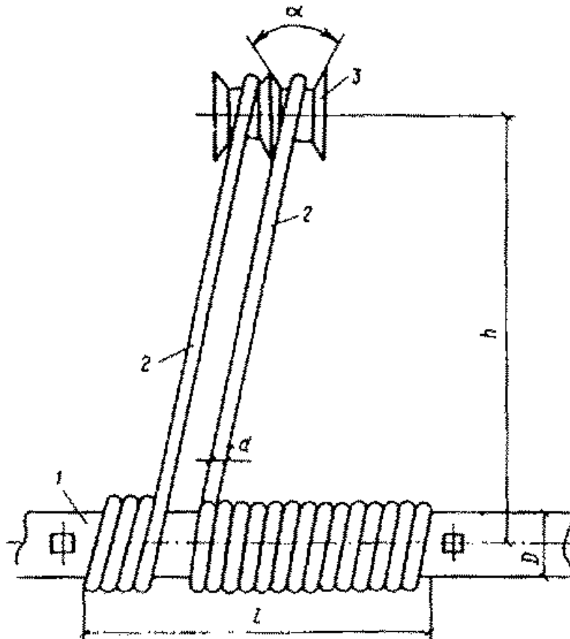
Рис. 9. Схема к расчету привода системы экранирования
