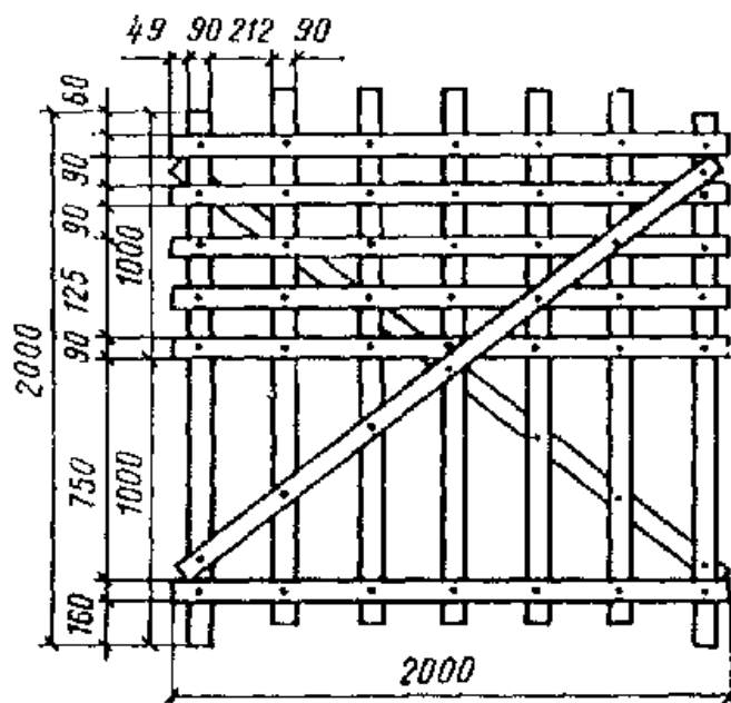
Рис. 26. Снеговой щит с разреженной обрешеткой
