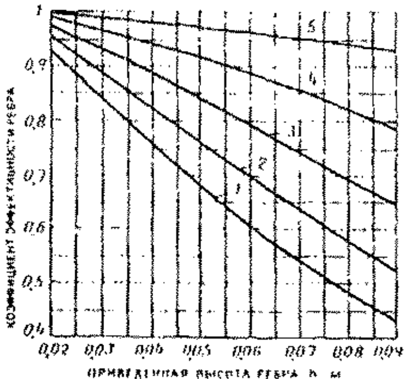
Рис. 20. График для определения коэффициента термической эффективности ребра m
