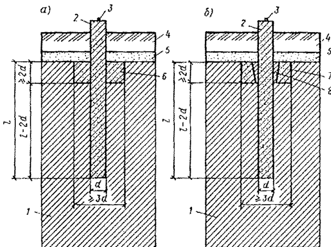
Рис. 2. Конструктивные решения фундаментов с шайбами
