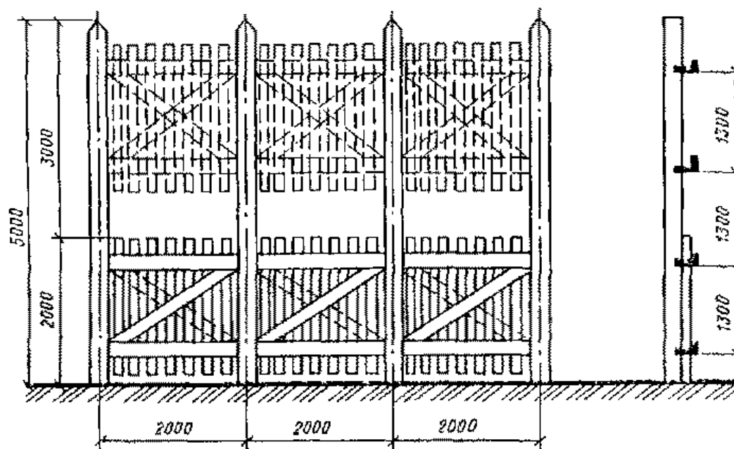
Рис. 30. Деревянный забор со съемными щитами
