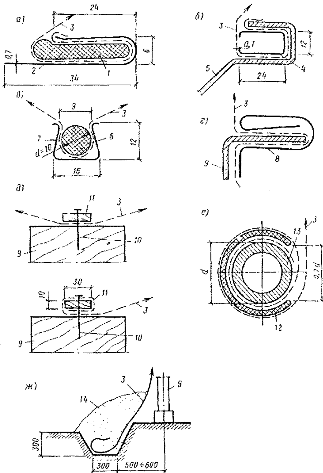
Рис. 4. Схемы рекомендуемых узлов крепления пленки к элементам каркаса теплиц
