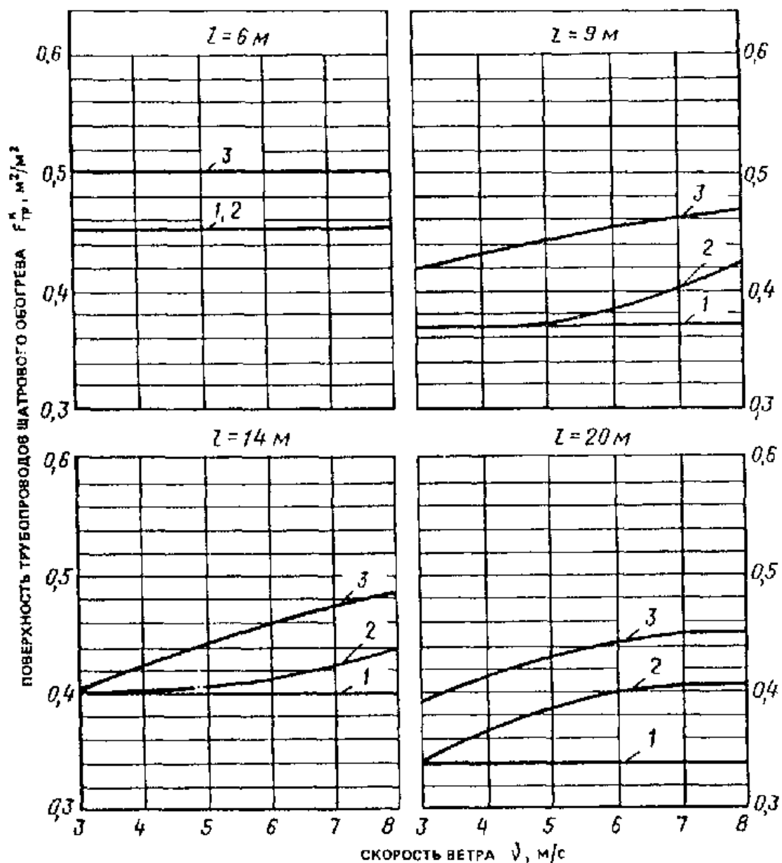
Рис. 23. Графики для определения требуемой поверхности трубопроводов шатрового обогрева при максимальной мощности калориферного обогрева и шаге трубопроводов подпочвенного обогрева S=0,4 м
