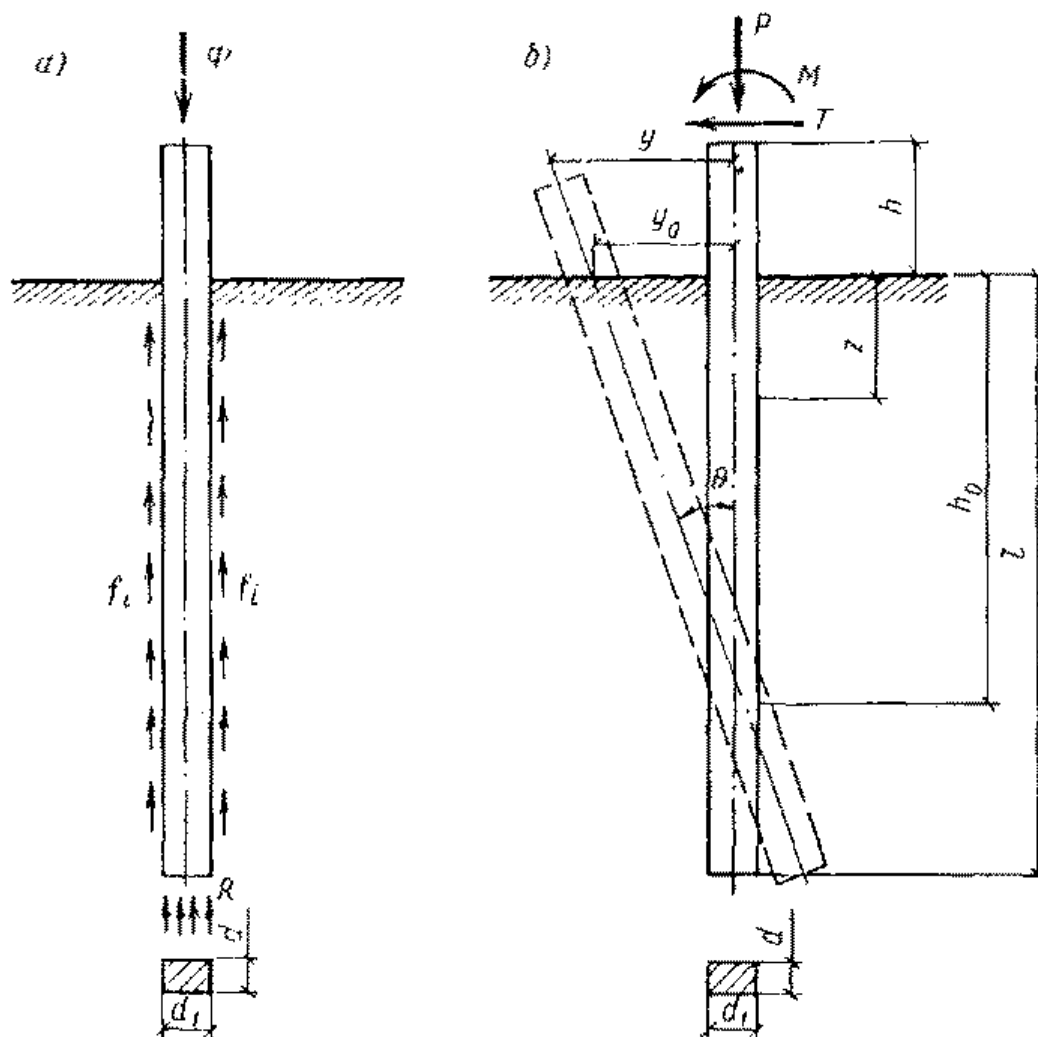
Рис. 3. Расчетные схемы микросвайных фундаментов теплиц
