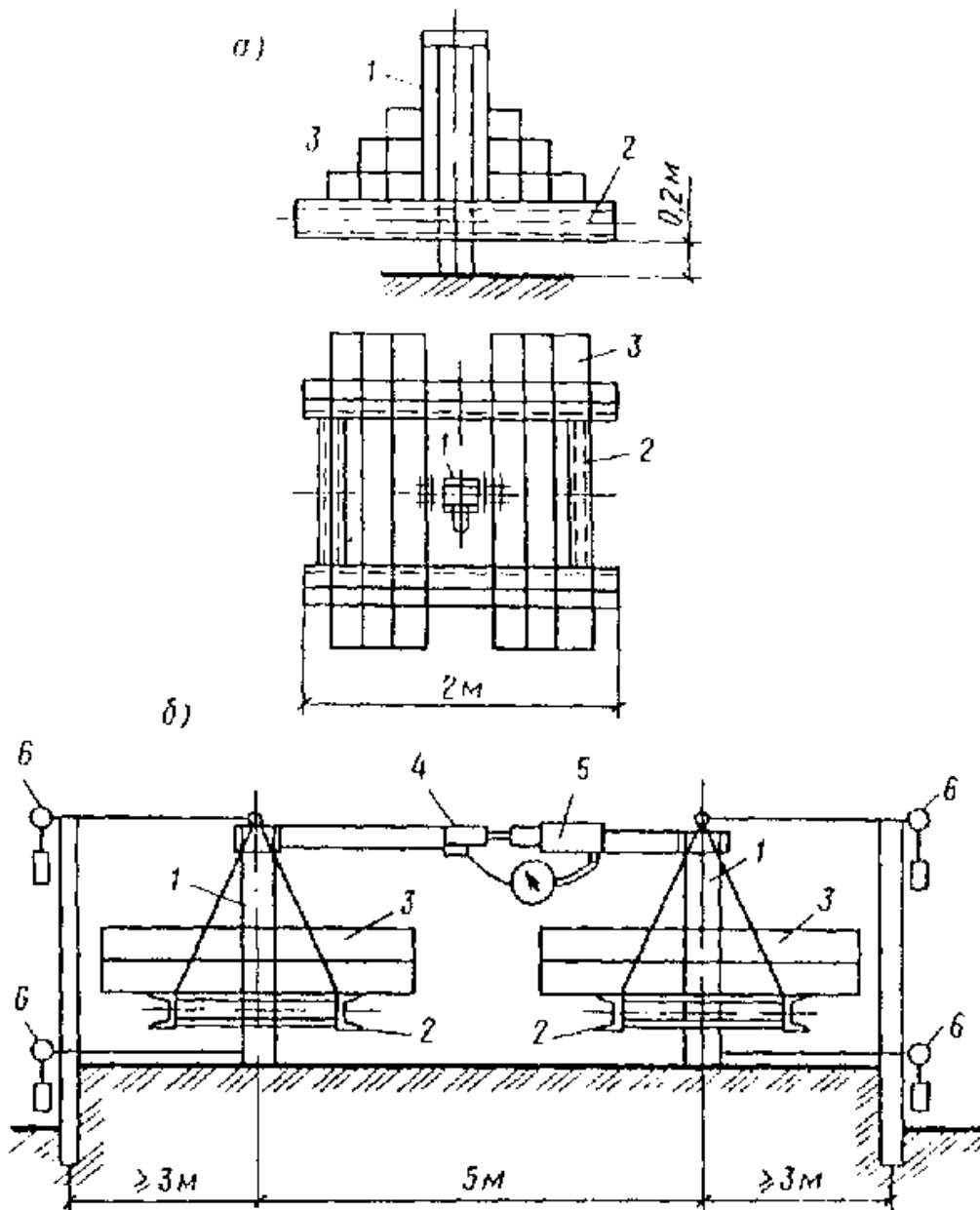
Рис. 1. Схемы загрузки свай
