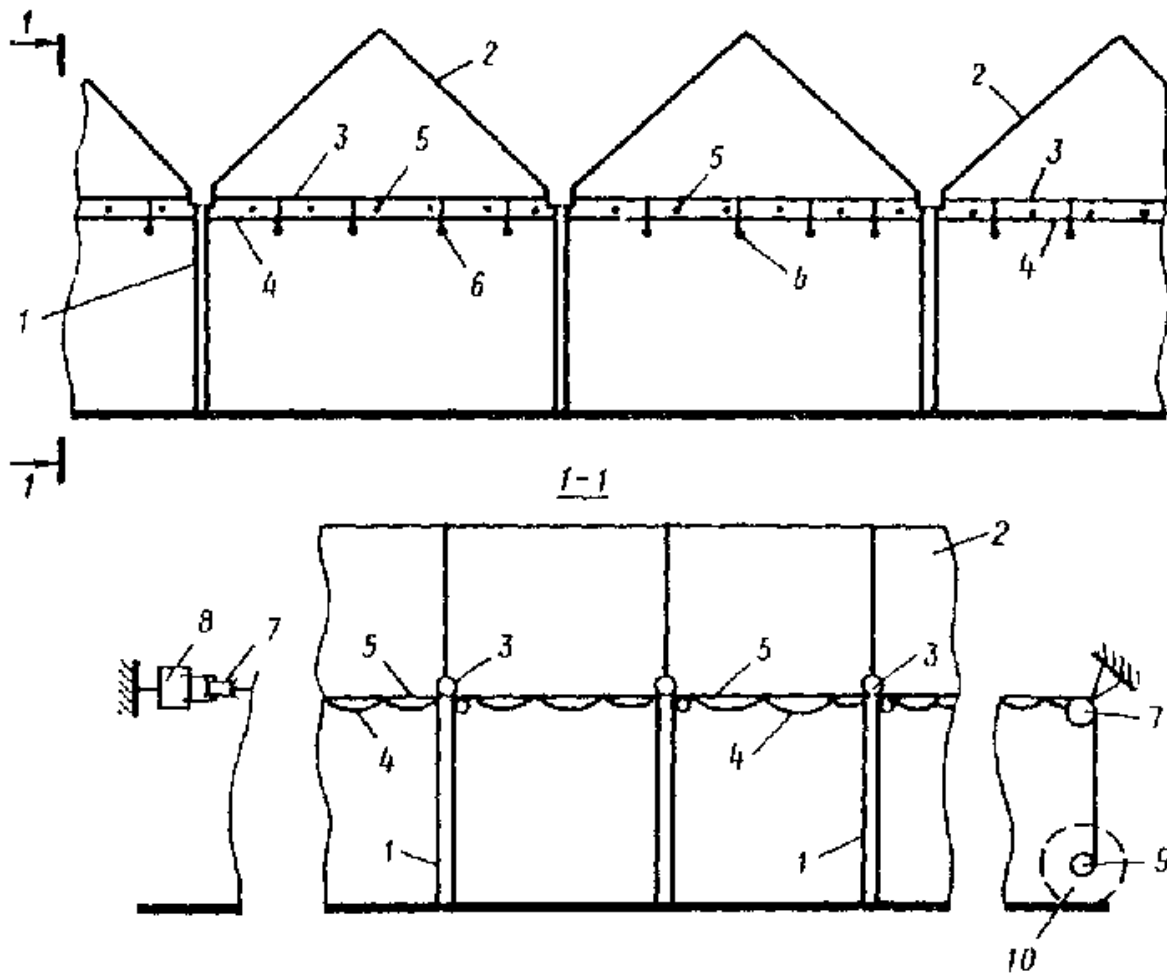
Рис. 7. Вариант схемы системы экранирования в многопролетной теплице
