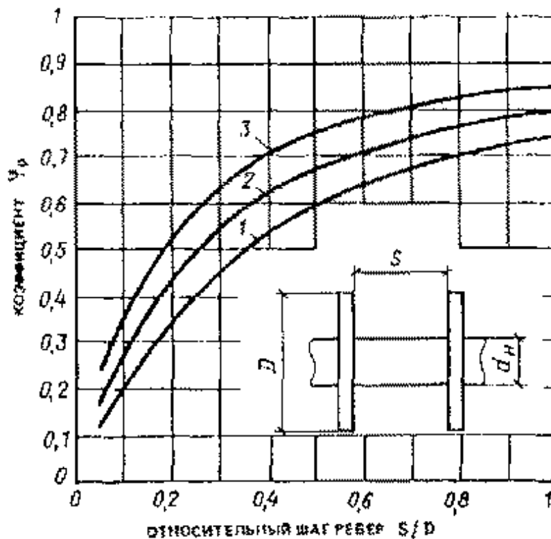
Рис. 18. График для определения коэффициента ф р
