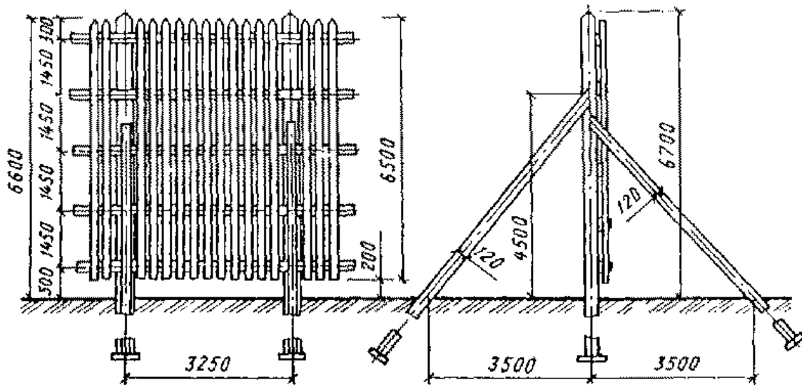
Рис. 28. Деревянный забор с нормальной обрешеткой
