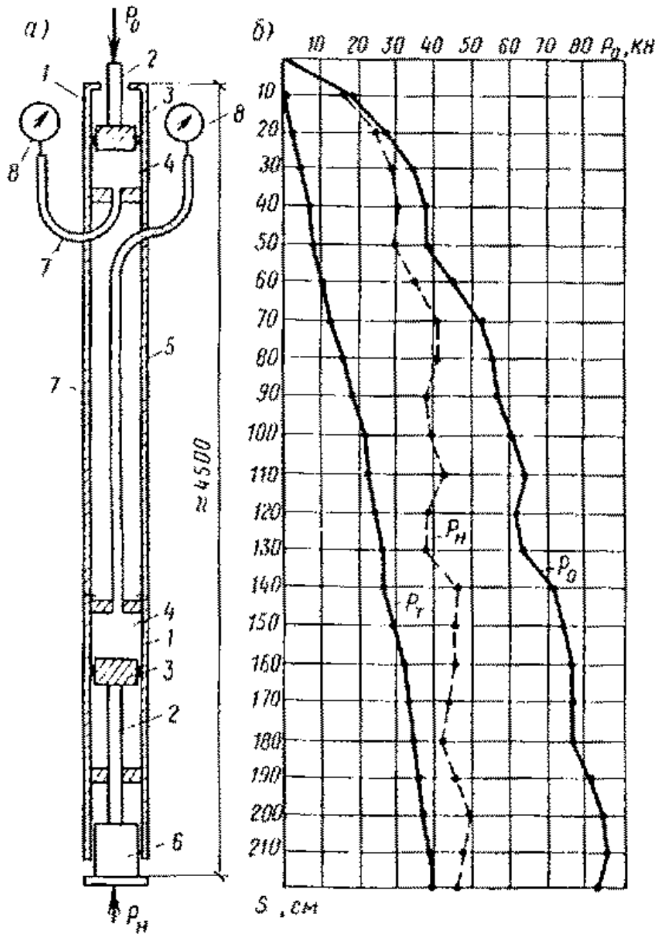
Рис. 4. Свая - штамп и ходограммы ее нагружения
