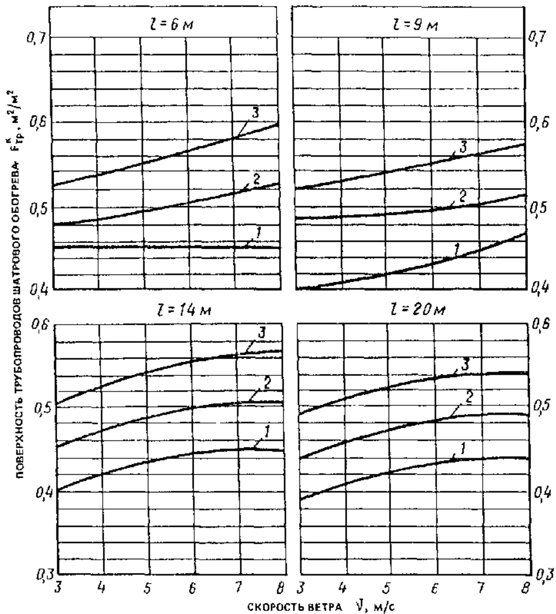
Рис. 22. Графики для определения требуемой поверхности трубопроводов шатрового обогрева при максимальной мощности калориферного обогрева и шаге трубопроводов подпочвенного обогрева S=1,5 м
