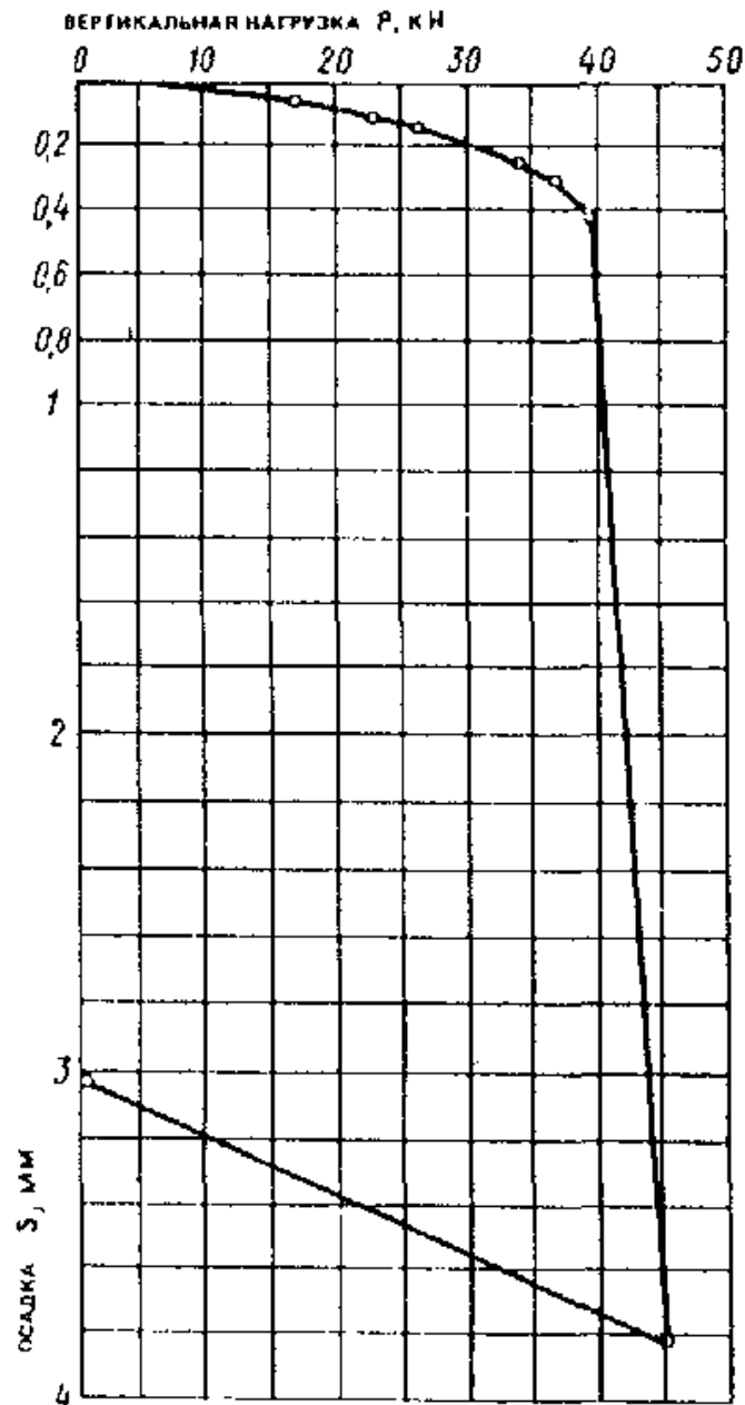
Рис. 2. График "осадка-нагрузка"
