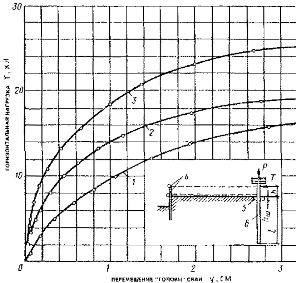
Рис. 3. Графики "нагрузка-перемещение"
