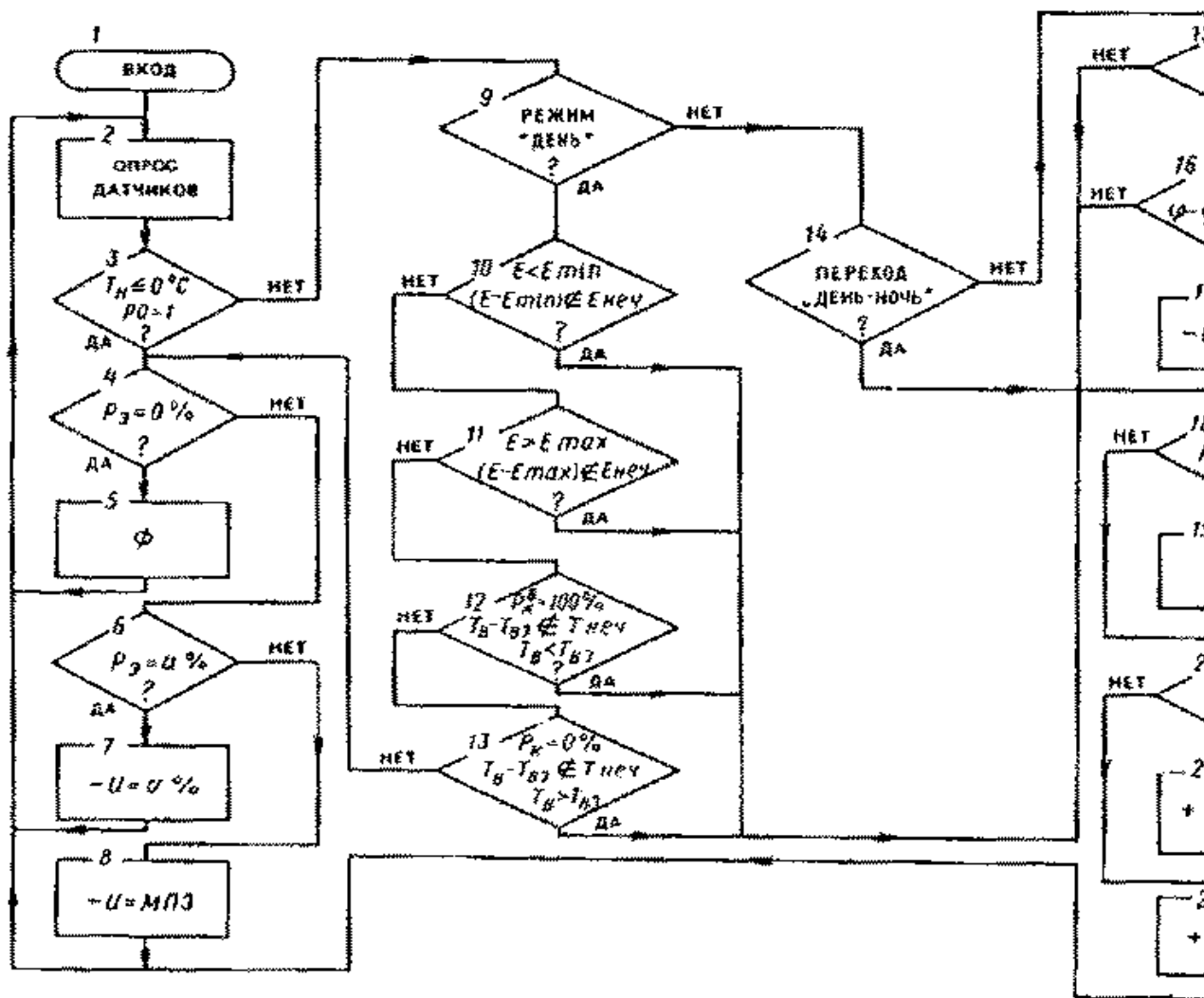
Рис. 11. Блок-схема алгоритма формирования управляющих воздействий о системе экранирования теплицы
