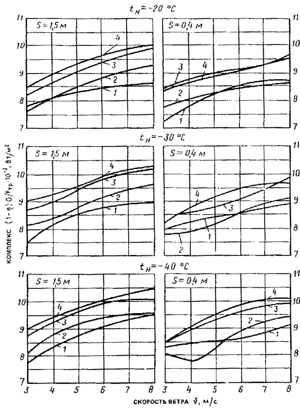
Рис. 24. Графики для определения максимальной мощности caloriferного обогрева \eta S - шаг трубопроводов подпочвенного обогрева, м; t_H - температура наружного воздуха; пролет теплицы; 1 - l=6 м; 2 - l=9 м; 3 - l=14 м; 4 - l=20 м
