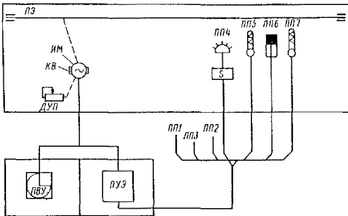
Рис. 10. Технологическая схема управления теплозащитным экраном
