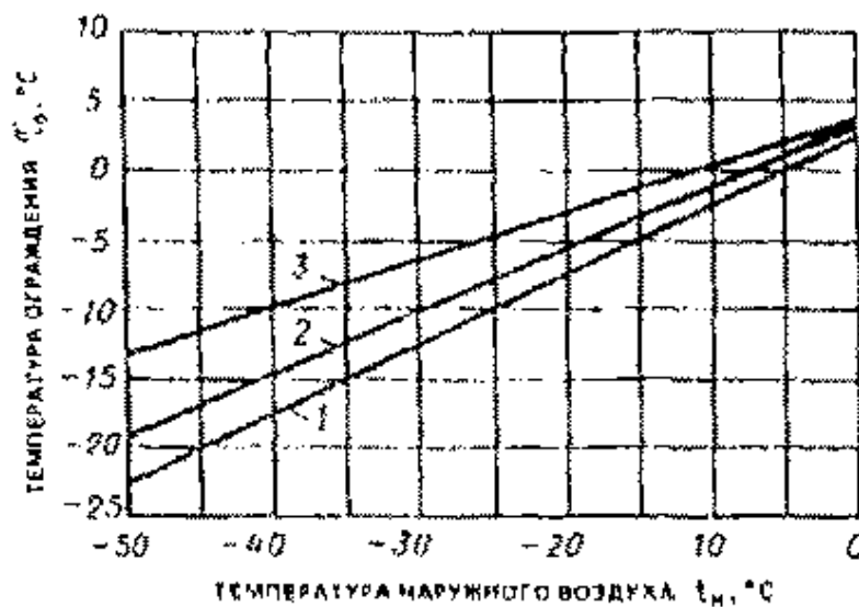
Рис. 19. График для определения температуры ограждений скорость ветра: 1 - v=1 м/с; 2 - v=6 м/с; 3 - v=3 м/с
