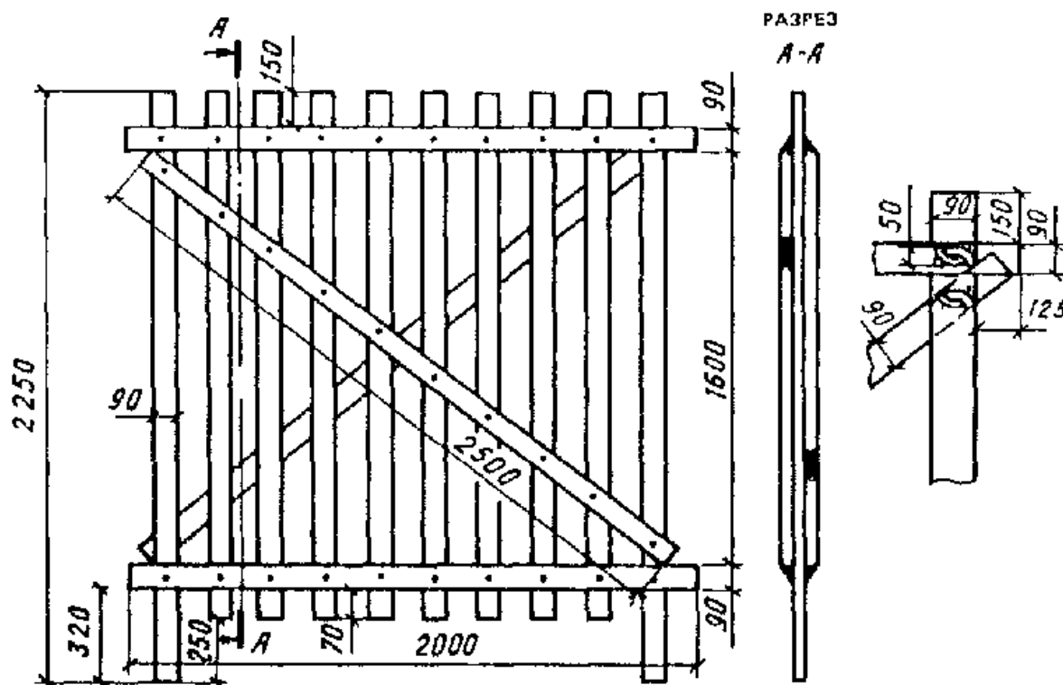
Рис. 25. Снеговой щит с нормальной обрешеткой
