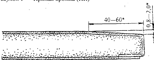
Рисунок 2 — Утоненная с лицевой стороны кромка (УК)
